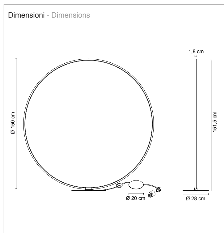
Completa di PUSH DIMM su cavo With PUSH DIMM on cable
